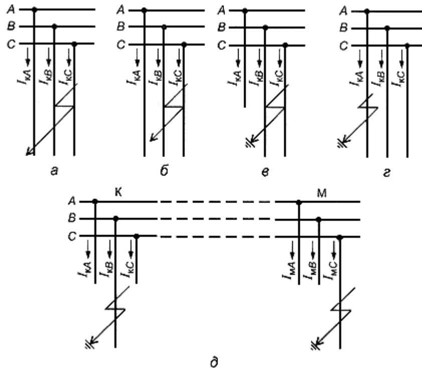
a - трехфазное КЗ-К (3) ; б - двухфазное КЗ-К (2) ; в - двухфазное КЗ на землю - К (1,1) ; г - однофазное КЗ на землю - К (1) ; д - двойное КЗ на землю - К (1-1)
